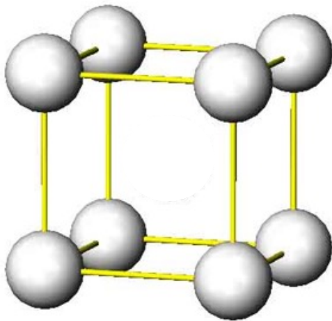
Cubique simple
