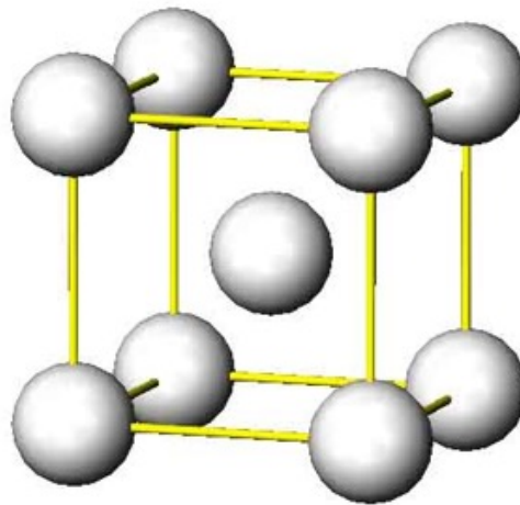
Cubique centré
